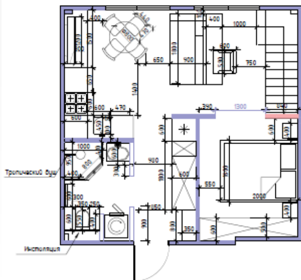
План расстановки оборудования на отм. +0,00 л с эргономическим анализом в размерах М1:50
