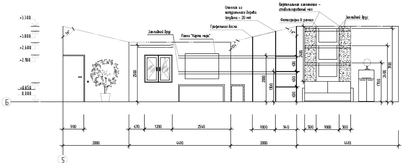
Развертка стен Кабинета
