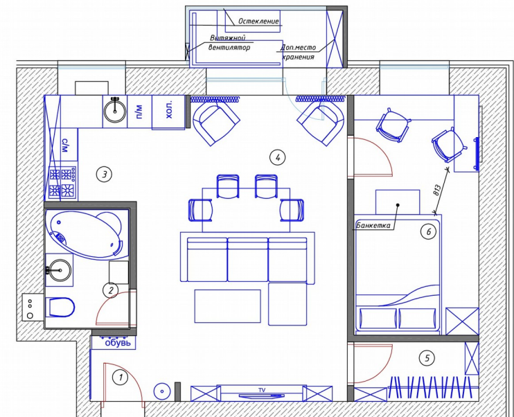
План расстановки мебели и оборудования
