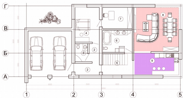
План расстановки оборудования на отм. 0,000
