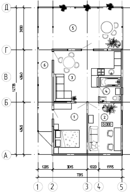
План с расстановкой оборудования
