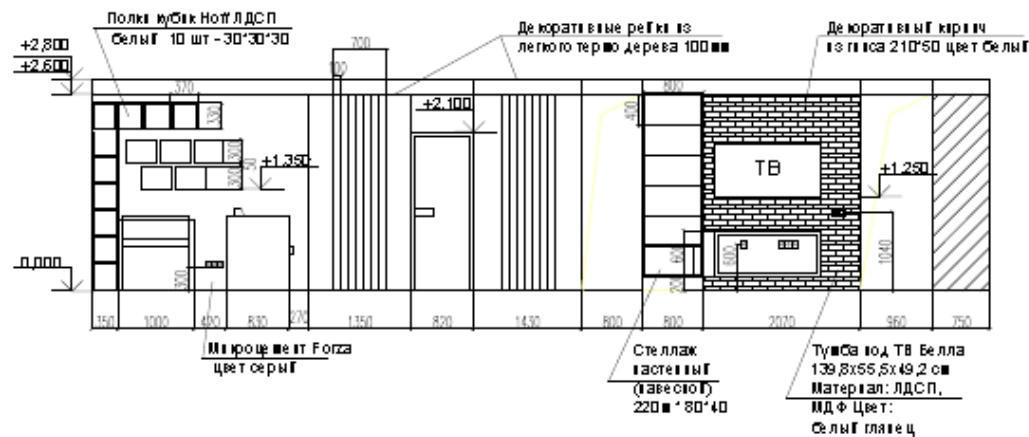
Развертки стен гостиной
